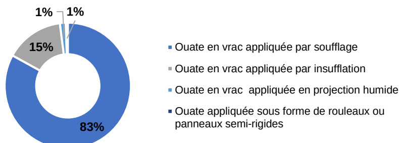
Figure 8. Mise en œuvre de la ouate de cellulose issue du papier
