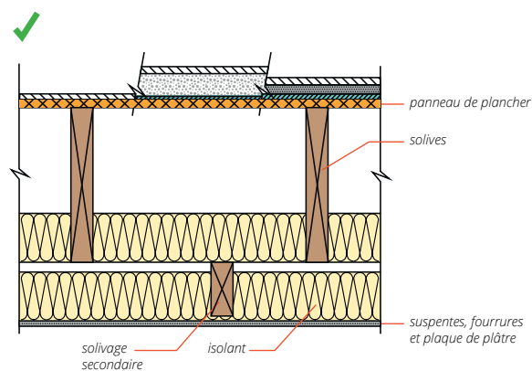
Schéma d'un plancher en double solivage bois massif qui permet d'avoir un système masse/ressort/masse et une désolidarisation des éléments (Source : http://www.catalogue-construction-bois.fr/sites/default/files/pi03-02.pdf ).
