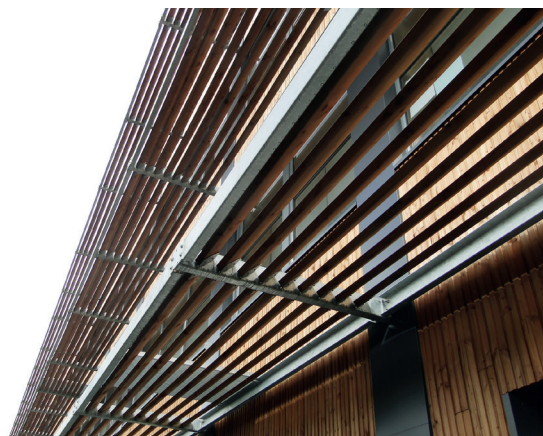
Exemple d'une solution corrective : installation de protections solaires pour limiter les apports solaires. ©AQC
