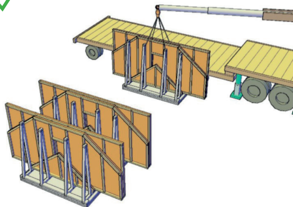
Exemple de colisage des panneaux ossature bois sur des racks modulables qui permettent de maintenir l'intégrité des panneaux (Source : « Façades ossatures bois non porteuses », RAGE, 2013 § 7.2.1).
