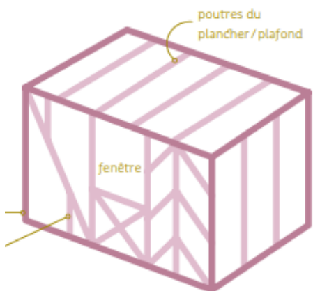
ossature secondaire "contreventement"
