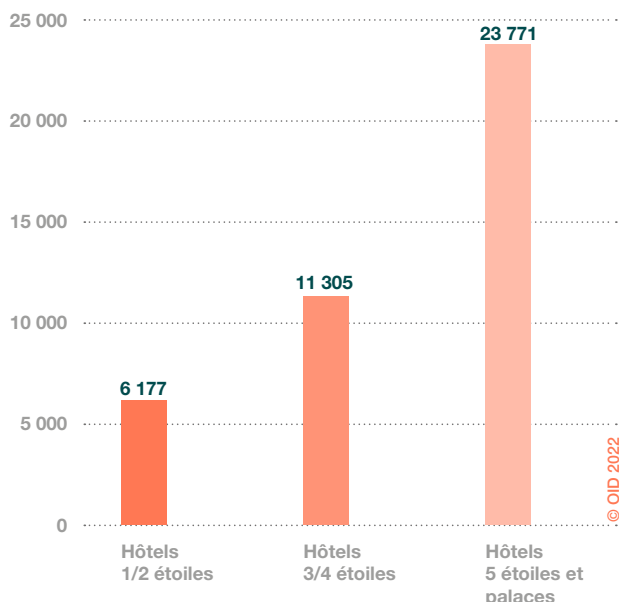
CONSUMMATION ÉNERGÉTIQUE RÉELLE PAR CHAMBRE EN ÉNERGIE PRIMAIRE SELON LE NIVEAU DE STANDING (en kWh EP /chambre.an)
