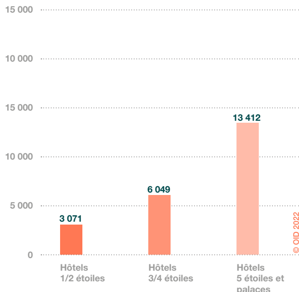
CONSUMMATION ÉNERGÉTIQUE RÉELLE PAR CHAMBRE EN ÉNERGIE FINALE SELON LE NIVEAU DE STANDING (en kWh EF /chambre.an)
