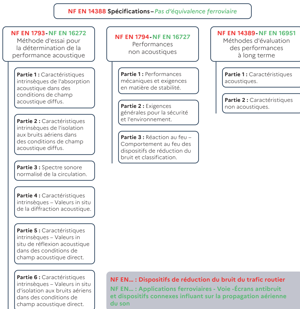
Figure 5 : Nomenclature des normes pour les dispositifs de réduction du bruit dans le cadre du bruit routier et ferroviaire
