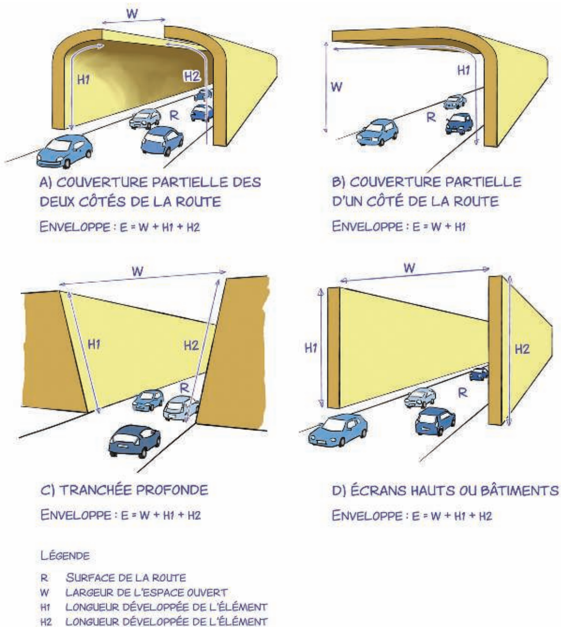
Figure 8 : Définition des conditions réverbérantes selon la configuration de l'infrastructure
