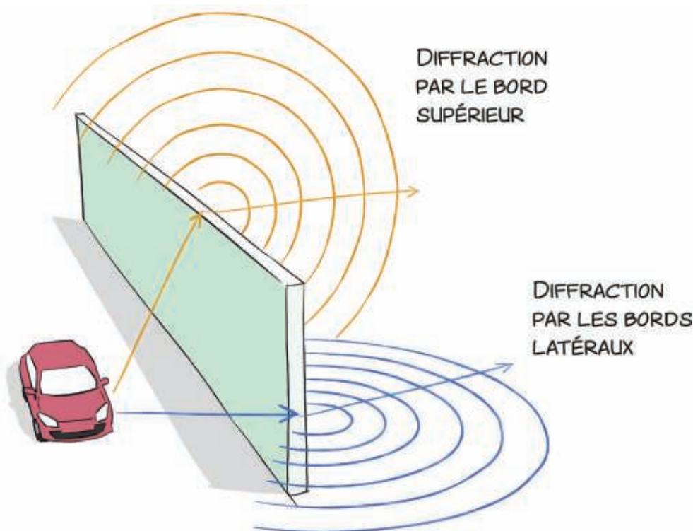
Figure 12 : Principe de la diffraction dans le cas d'un écran acoustique
