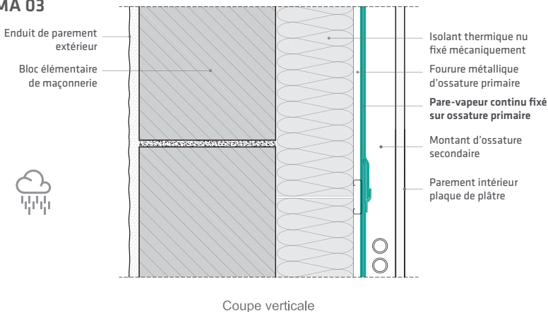
Coupe verticale
