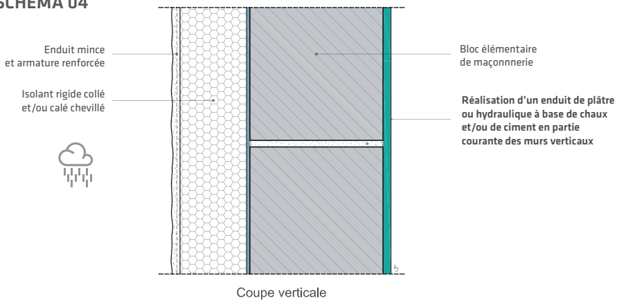
Coupe verticale
