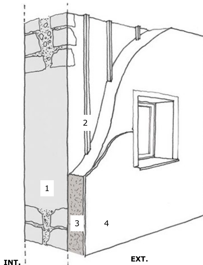
INT. EXT. Axonométrie écorchée de la pose d'un enduit isolant en ITE - © SHA
