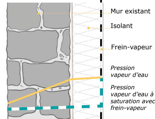
Schéma de migration de la vapeur d'eau – avec frein-vapeur – © Ajena
