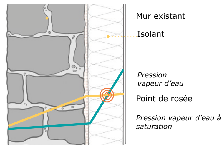
Schéma de migration de la vapeur d'eau – sans frein-vapeur et avec point de rosée – © Ajena
