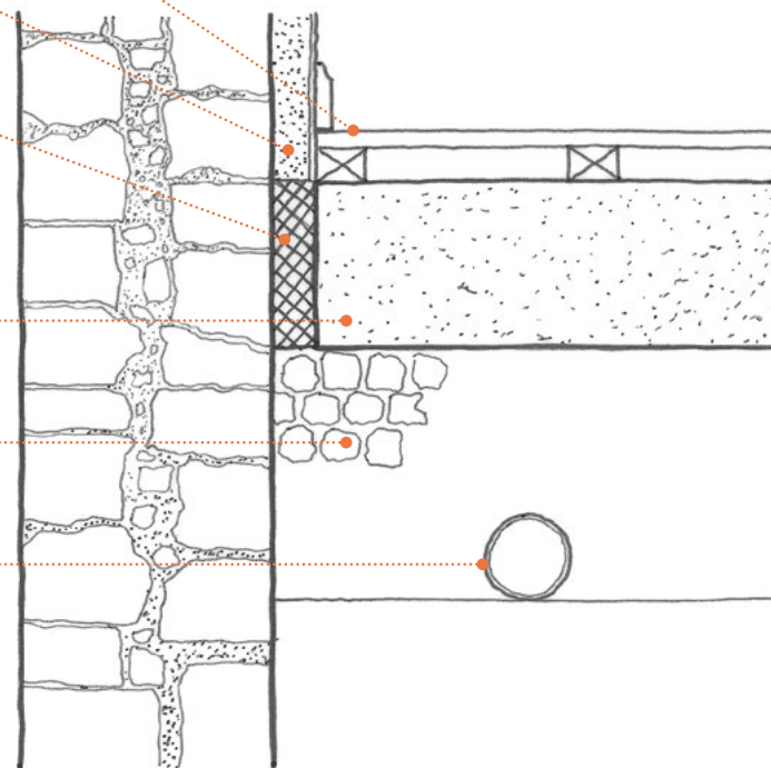
Coupe sur plancher bas – © SHA
