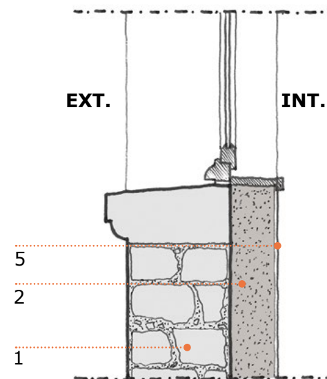
Détail appui de fenêtre © SHA
