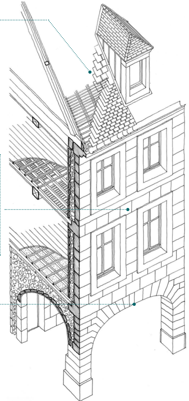
Encadrement de baies en pierre de taille
