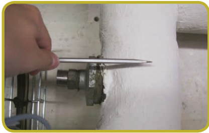
Le doigt de gant atteint le centre de la canalisation, l'élément sensible de la sonde sera bien placé dans l'écoulement
