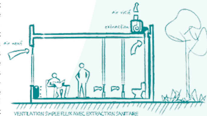
Figure 17 : Ventilation simple flux avec extraction sanitaire dans un immeuble tertiaire.
