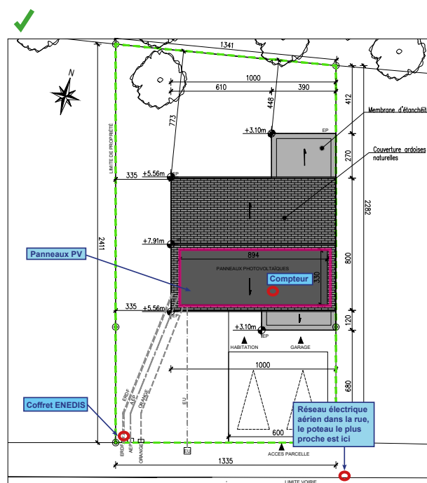
Plan de masse 1/100°
